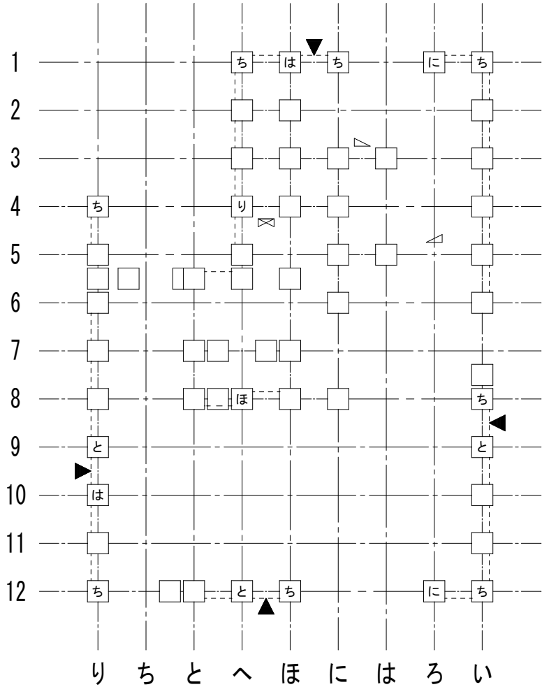
1 階柱壁伏図
