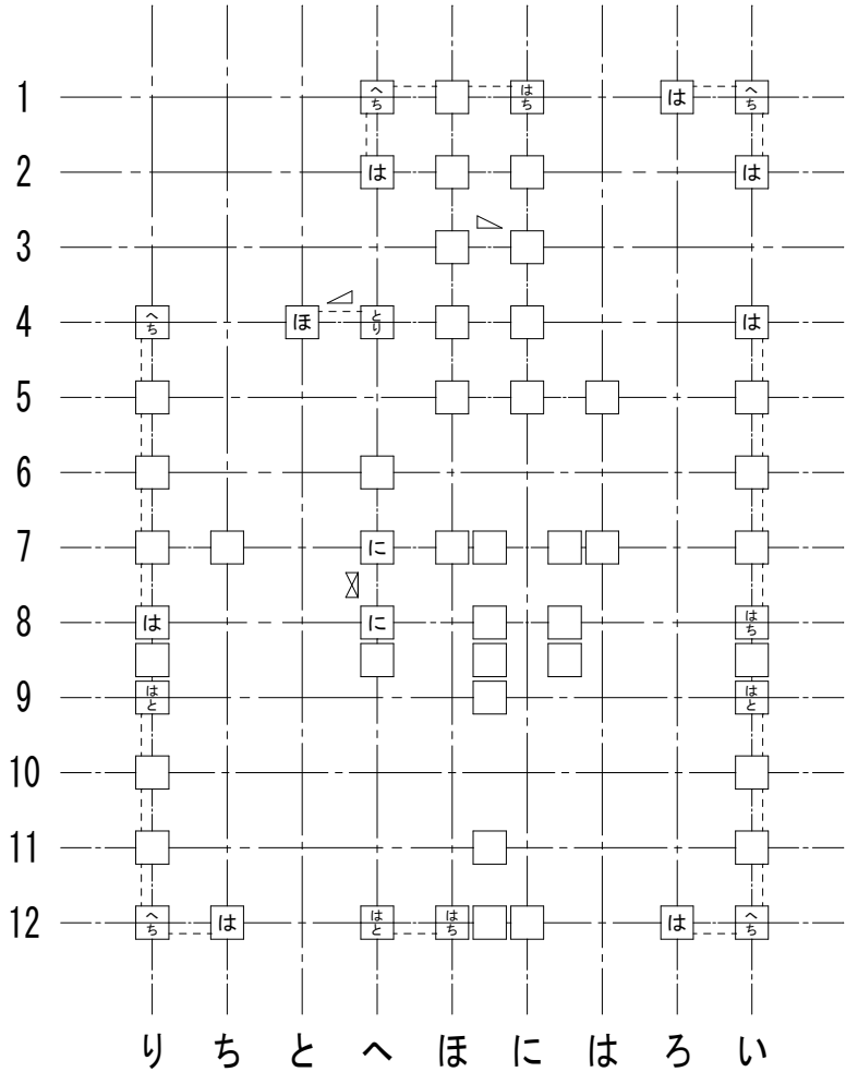
2 階柱壁伏図
